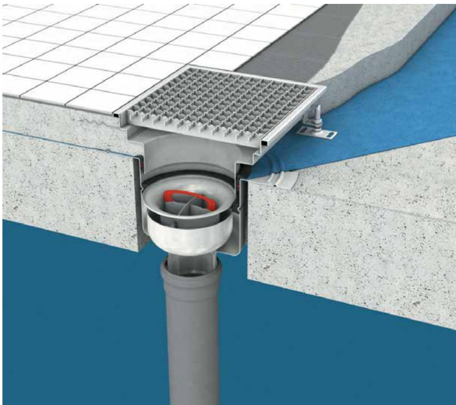
Primer odvodnjavanja v medetažni konstrukciji s požiralnikom s tlačno prirobnico.
