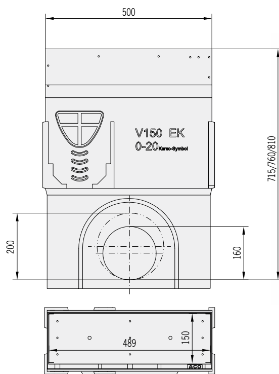
SlotTop 150 iztočni element (zbiralnik Multiline V 150 s SlotTop revizijskim elementom), dolžine 50 cm
