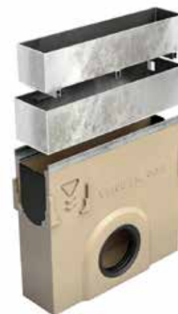
SlotTop 100 iztočni element (zbiralnik Multiline V 100 s SlotTop revizijskim elementom), dolžine 50 cm
