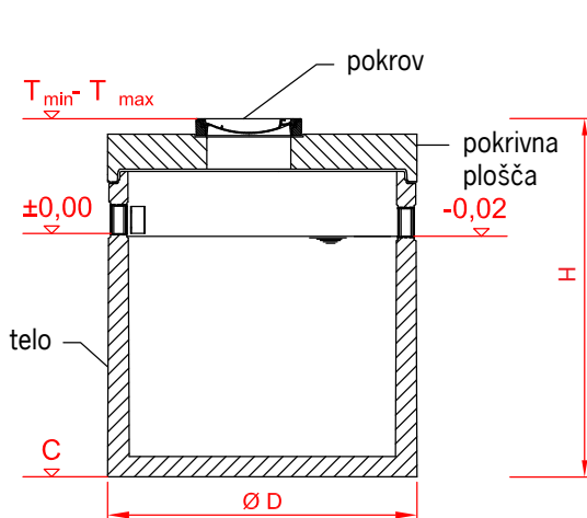
Usedalnik SF (osnovna izvedba)
