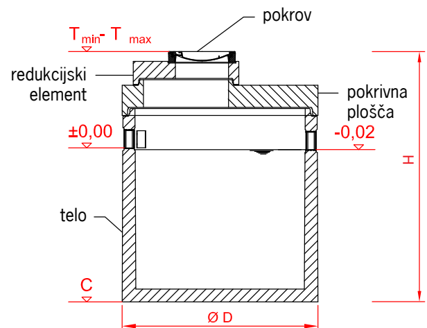
Usedalnik SF (izvedba za povišanje)
