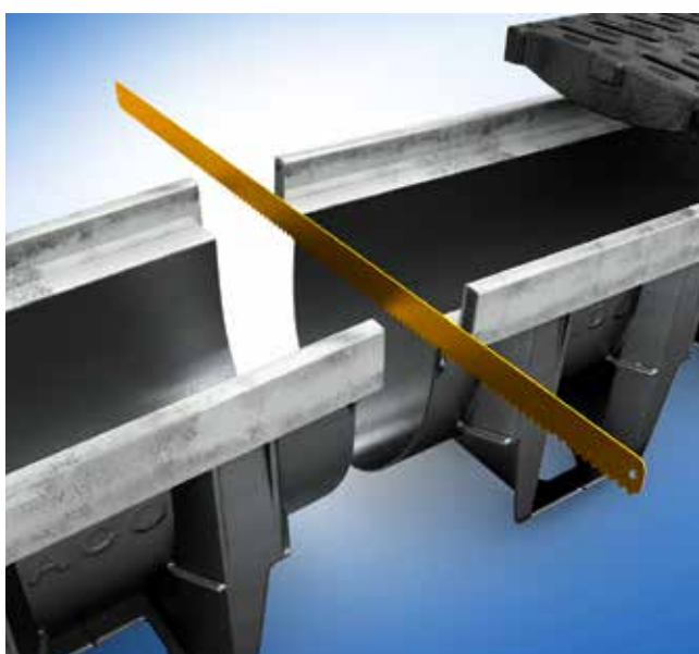
Kanaleta dolžine 50 cm dobimo tako, da z ročno žago na označenem mestu in po vodilu prerežemo kanaleta dolžine 100 cm
