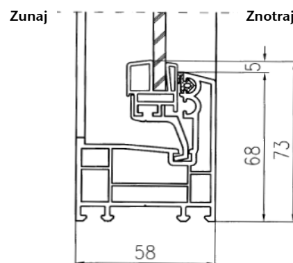
Prerez kletnega okna ACO Markant
