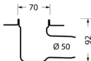
Horizontalna prirobnica
