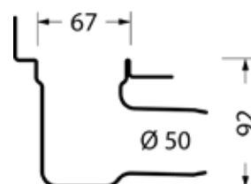
Stenska prirobnica
