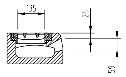
Prerez A-A
