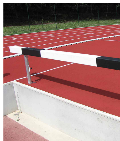
Kompleten element-ACO SPORT 8100 bazen za vodo za tek na 3000 m z ovirami
