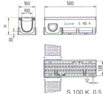
S 100 K, 0.5 M
