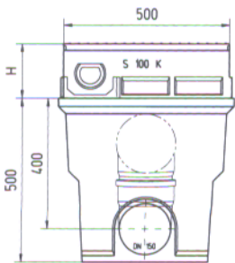
S 100 K, zbiralnik dolga izvedba
