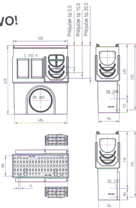
S 150 K enodelen zbiralnik z iztokom DN 150 ali DN 200
