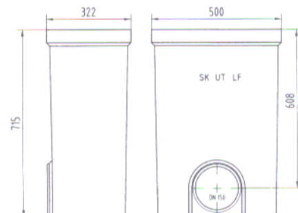
S 200 K, zbiralnik spodnji del, dolga izvedba z iztokom DN 150 ali DN 200
