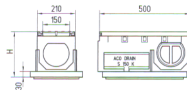
S 150 K, zbiralnik zgornji del
