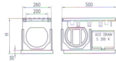
S 200 K, zbiralnik zgornji del
