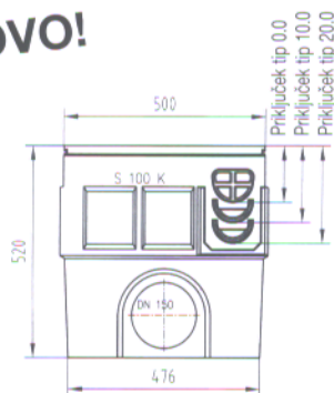
S 100 K, enodelen zbiralnik, z iztokom DN 100 ali DN 150
