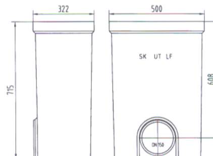
S 150 K, zbiralnik spodnji del, dolga izvedba z iztokom DN 150 ali DN 200
