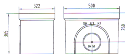
S 150 K, zbiralnik spodnji del, kratka izvedba z iztokom DN 150 ali DN 200
