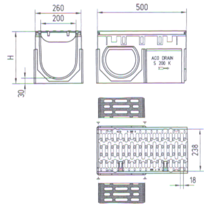
S 200 K, 0.5 m
