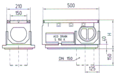
S 150 K, 0.5 m z vgrajenim iztokom DN 150 s tesnilom
