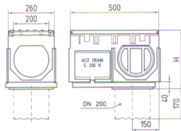
S 200 K, 0.5 m z vgrajenim iztokom DN 200 s tesnilom
