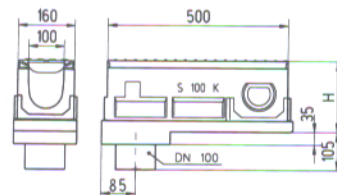
S 100 K, kanaleta z vgrajeno varnostno loputo DN 100
