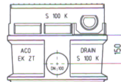
S 100 K, zbiralnik kratka izvedba, spodnji del se lahko uporabi tudi kot vmesni del
