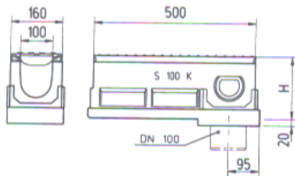
Kanaleta S 100 K, 0.5 m z vgrajenim iztokom DN 100 s tesnilom
