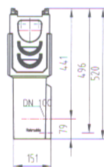
S 100 K, enodelen zbiralnik, z iztokom DN 100 ali DN 150
