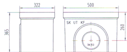
S 200 K, zbiralnik spodnji del, kratka izvedba z iztokom DN 150 ali DN 200
