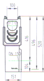
S 100 K, enodelen zbiralnik, z iztokom DN 100 ali DN 150
