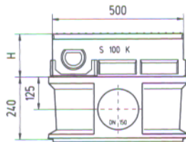
S 100 K, zbiralnik kratka izvedba, spodnji del se lahko uporabi tudi kot vmesni del
