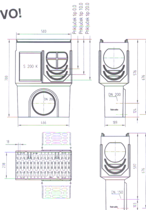
S 200 K enodelen zbiralnik z iztokom DN 150 ali DN 200
