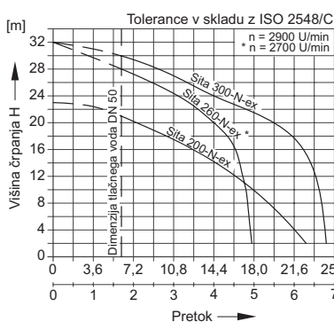
Črpalni diagram
