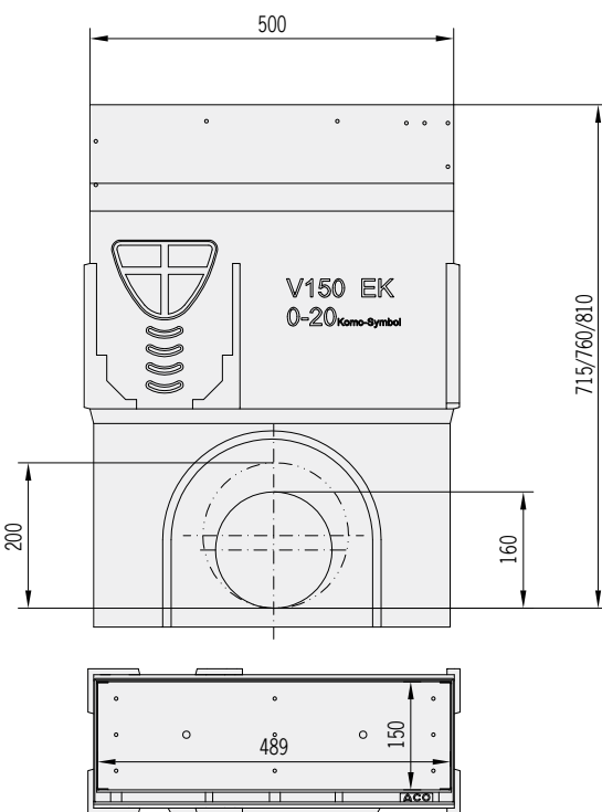
Slotline 150 iztočni element (zbiralnik Multiline V 150 s SlotTop revizijskim elementom), dolžine 50 cm
