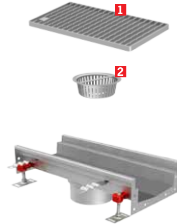
Kanalete Modular 125 / 20
