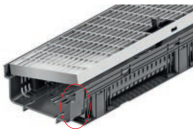
ACHTUNG! Vor Verlegen des ersten Rinnenelements die Rinne am Rinnenanfang um 1 cm kürzen – siehe Schnittführung ○
