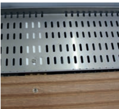
Verschraubung des Rinnenkörpers durch die 4-mm-Dränschlitzte im Rinnenboden
