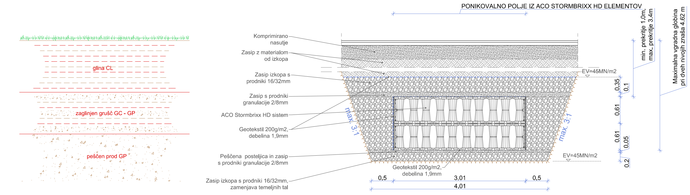
PREČNI PREREZ PONIKOVALNEGA POLJA PP1
