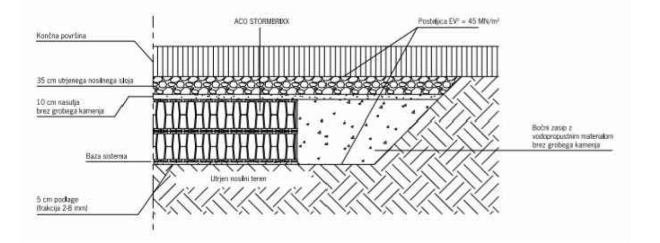
ACO STORMBRIXX SD ELEMENTI:
