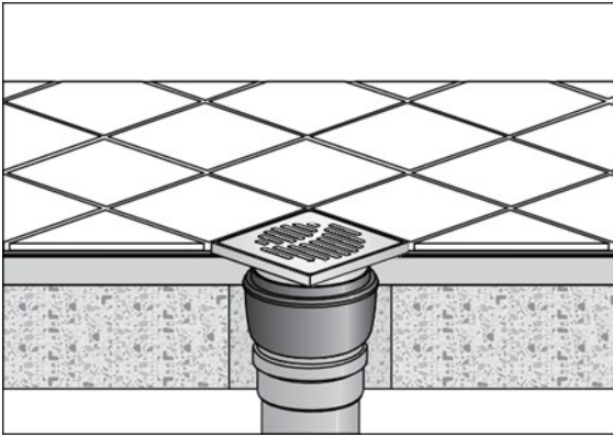
Primer 1: Vgradnja brez prirobnice
