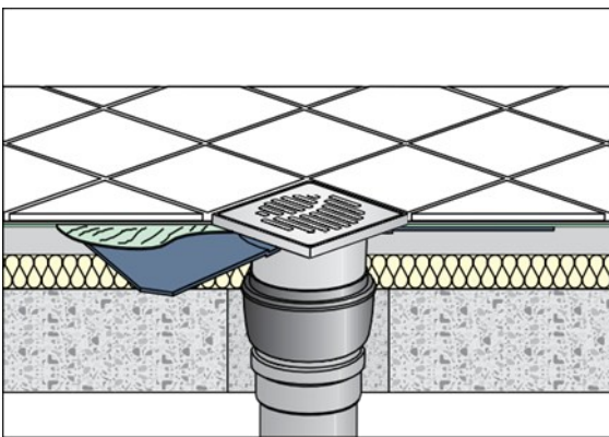
Primer 2: Vgradnja s tankoslojno prirobnico
