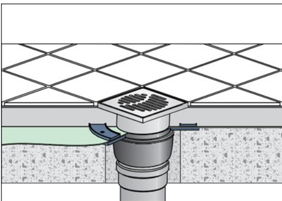
Primer 3: Vgradnja s tlačno prirobnico
