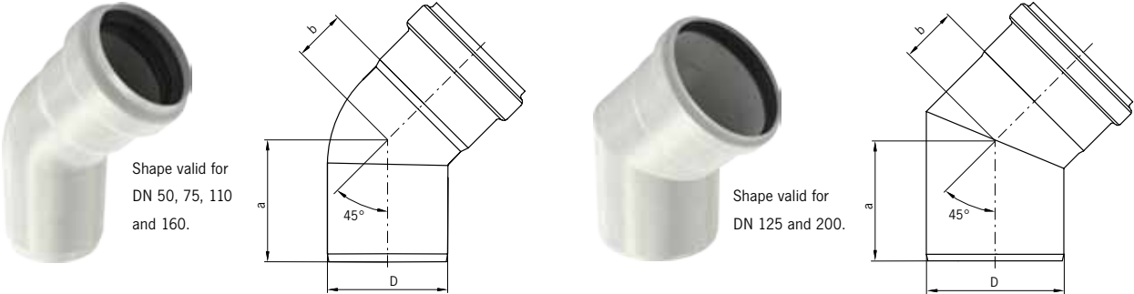
AP bend 45°
