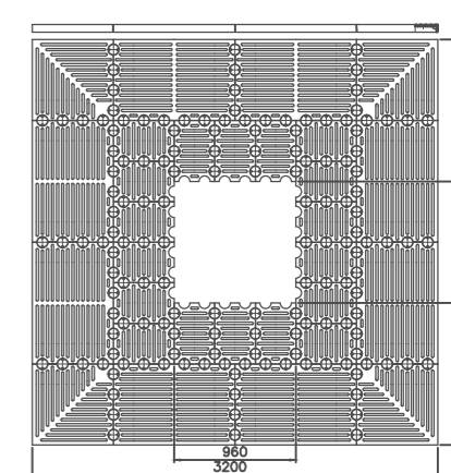
Drevesna rešetka WOTAN kvadratna Tip 324 Dimenzije (mm) zunanja 3200/3200, odprtina 960/960
