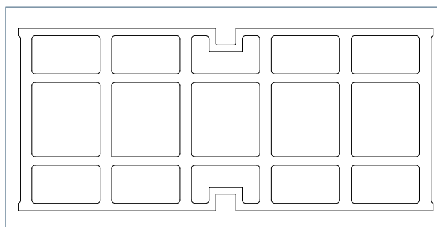
Standardna osnova nazivne širine 200 (500 x 223 mm)
